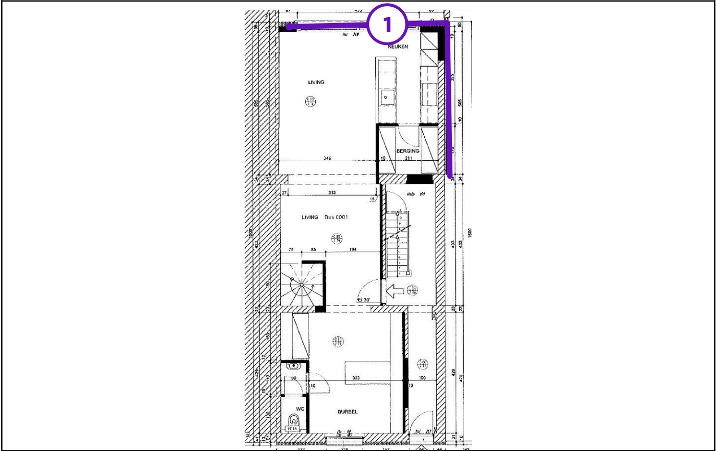
Legende van plan 1.2: inkom- en trappenhall gelijkvloers
